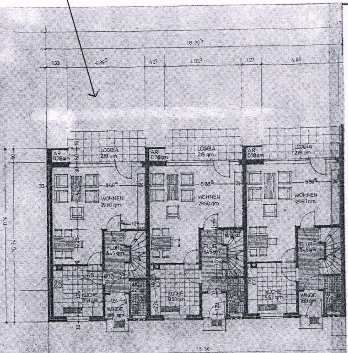
ERDGESCHOSS
