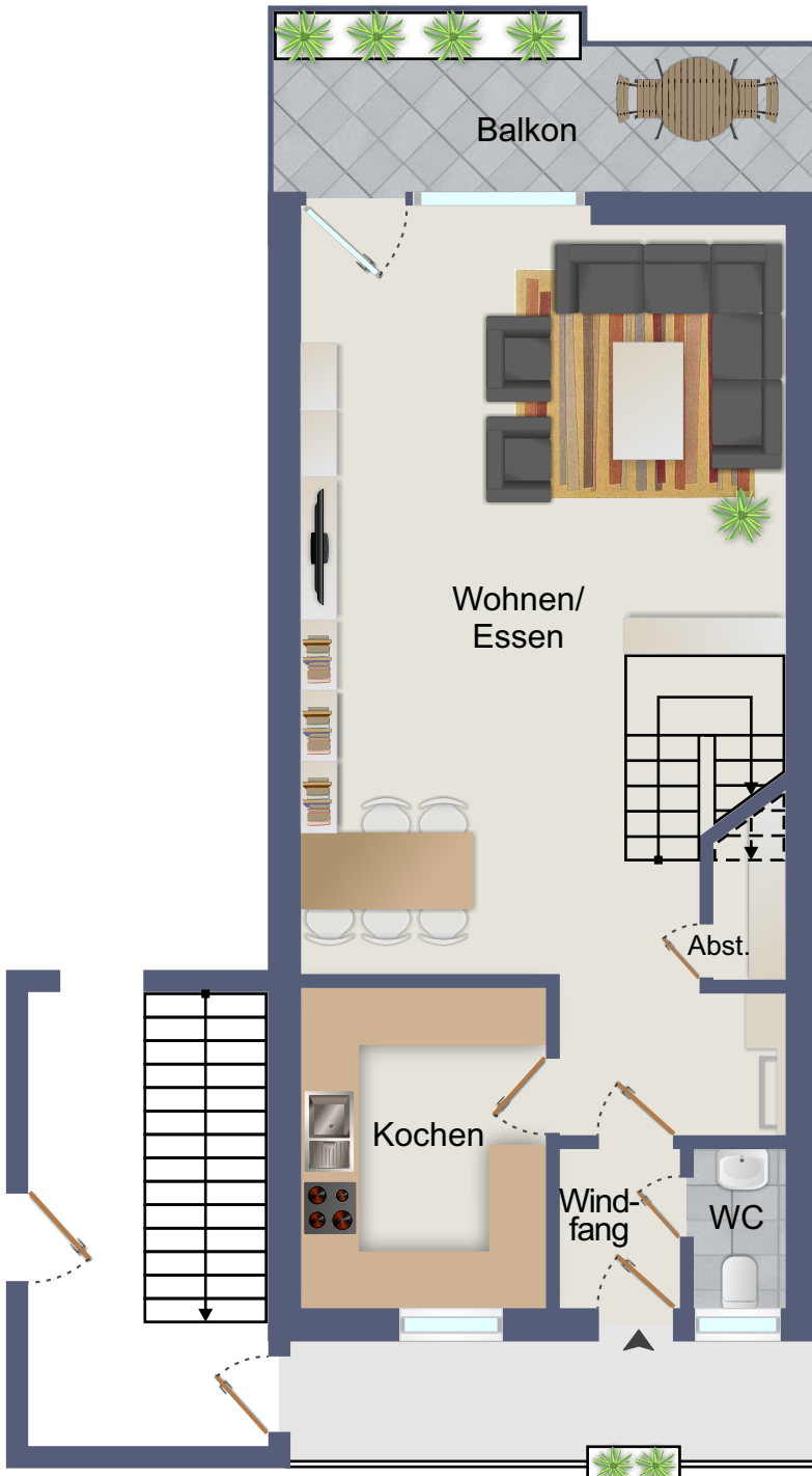
1.2. Obergeschoss , Aktueller Zustand
